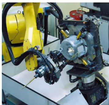
Öntvény megmunkáló robot
